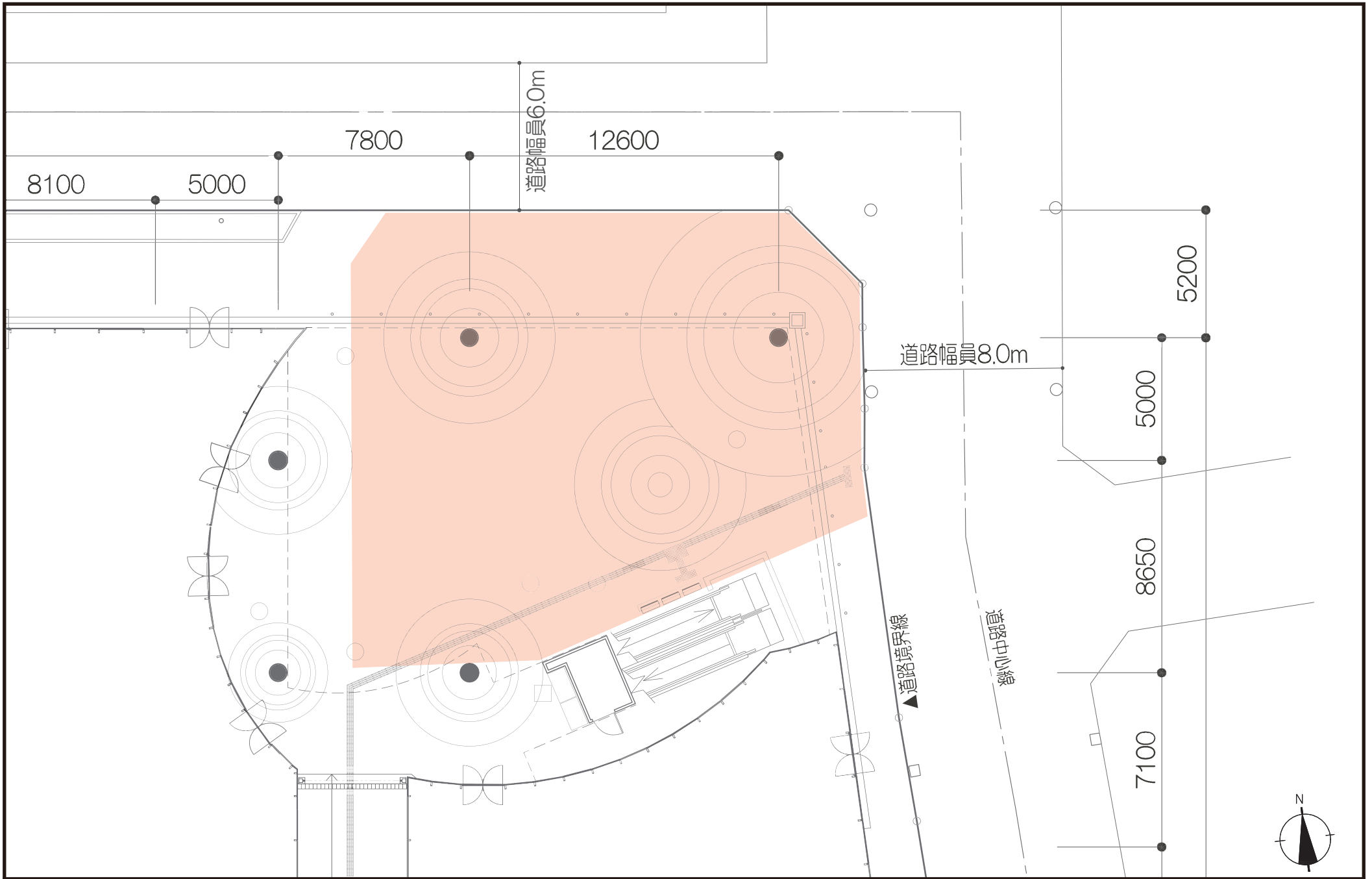
柳ヶ瀬グラスル35 1階平面図 1/200
